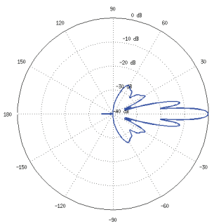
H-Plane
